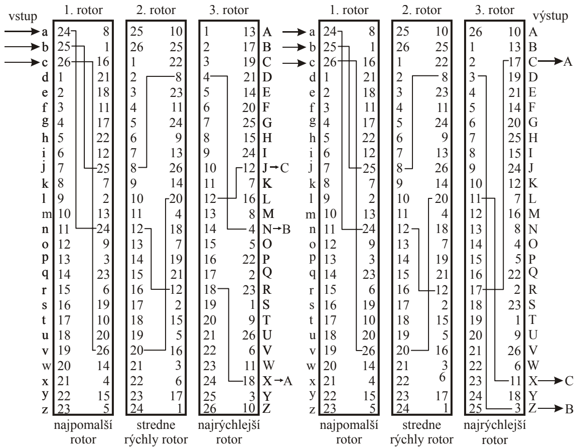
Obr. 2.6 Princíp rotorového stroja s tromi rotormi
