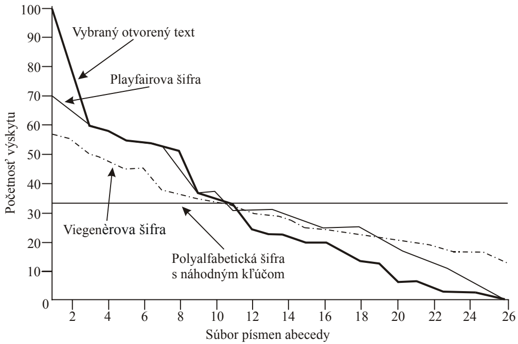
Obr. 2.5 Frekvenčná distribúcia písmen zašifrovaného textu pre rôzne typy šifier
