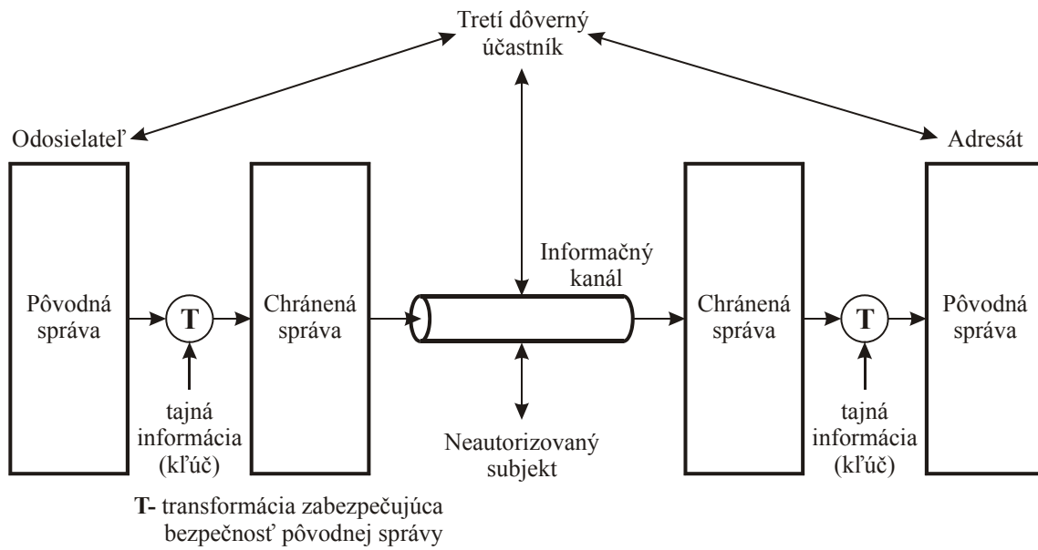
Obr. 1.3 Model sieťovej bezpečnosti
