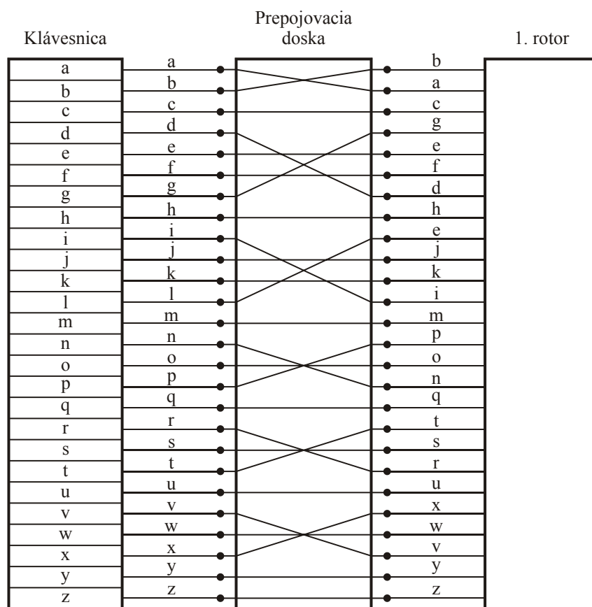
Obr. 2.7 Prepojovacia doska a jej funkcia
